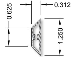
Trapezoidal 990853/990871
