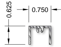
Frame Filler 999412
