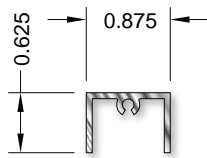
Frame Filler 999402
