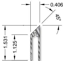
45° Beveled Filler 990854
