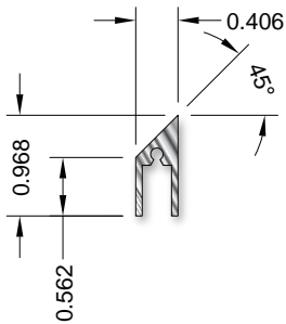
45° Beveled Filler 990763
