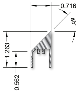
45° Beveled Filler 990883
