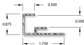
1/2" Drywall Trim (No Clip) 999438
