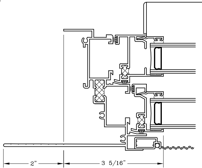
2" Flange Frame (Jamb Shown)
