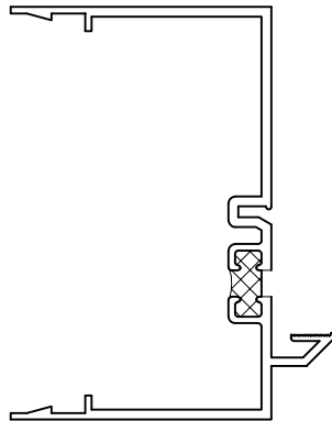
.062 Wall Extended Leg Jamb
