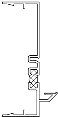
.062 Wall Jamb
