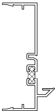
.080 Wall Jamb
