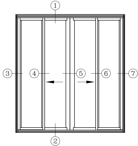
ELEVATION OXXO - Shown
